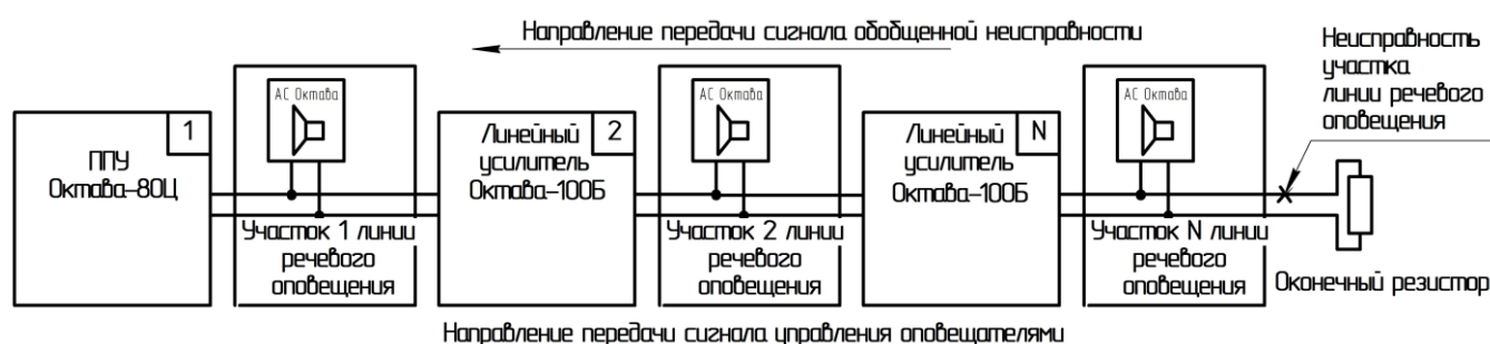
Рисунок 1.4 - Схема передачи сигнала «Неисправность» по линии речевого оповещения
