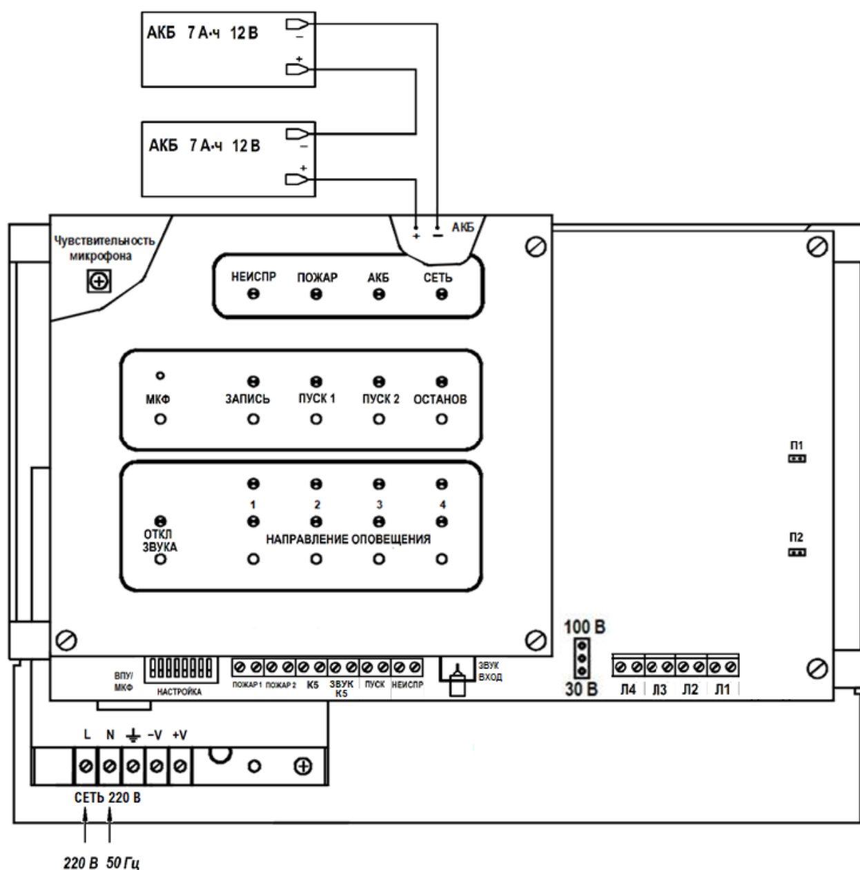
Рисунок 1.2 - Плата ППУ
